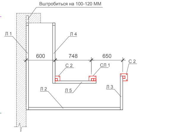
Разрез 2-2
