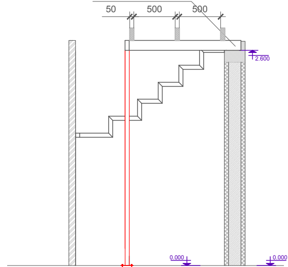
Разрез 2-2
