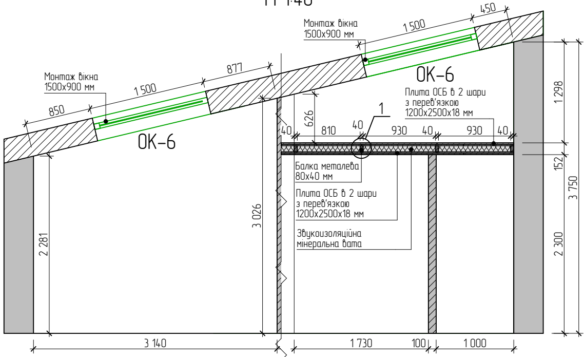
Розріз 1-1 М 1:40
