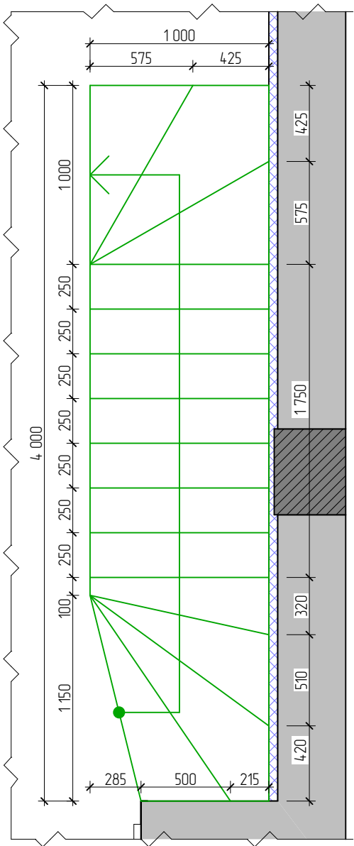
Фрагмент плану № 1 М 1:30
