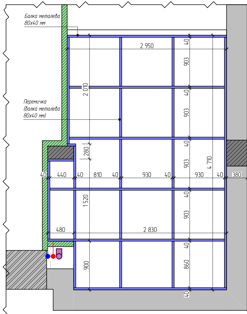
План монтажу балок
