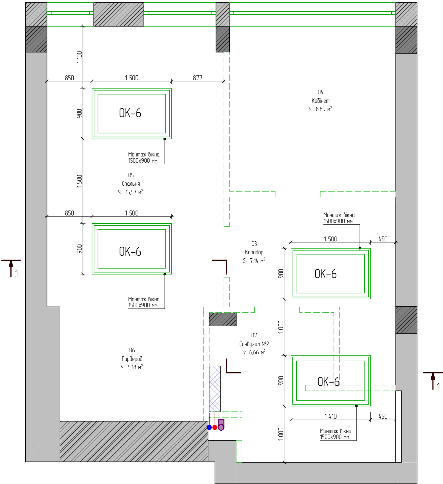
План монтажу вікон в перекритті
