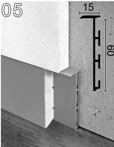
Плінтус прихованого монтажу Р-105.. 60x15x2500
