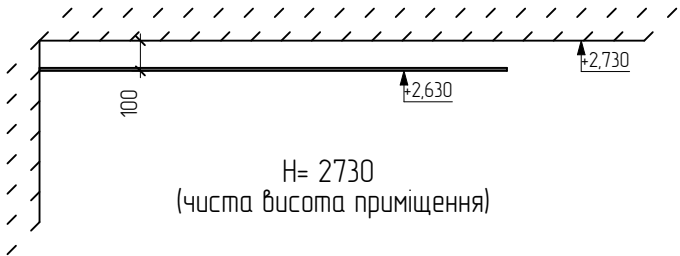
Січення тиньової стелі
