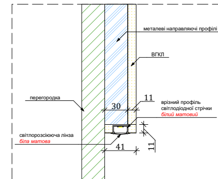
Вузол №2
