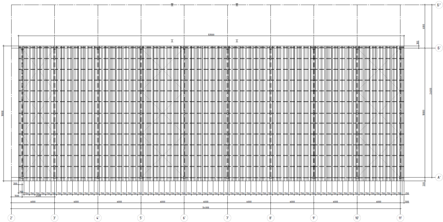
Схема розташування настилу Н57-0.7-750
