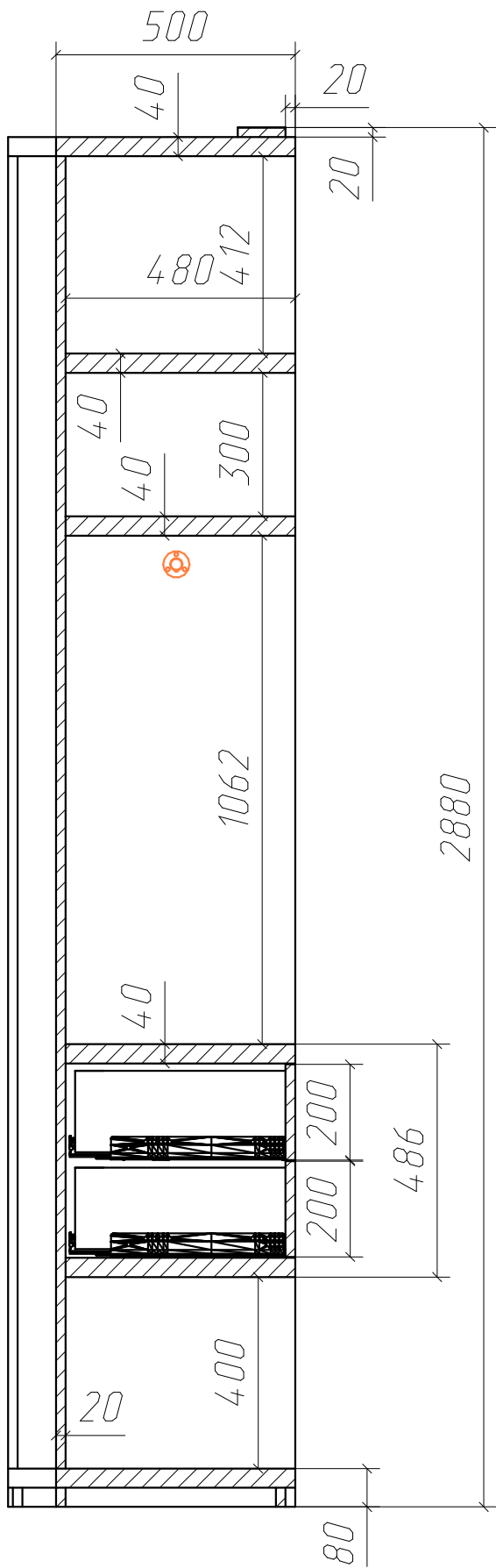
Сечение В-В
