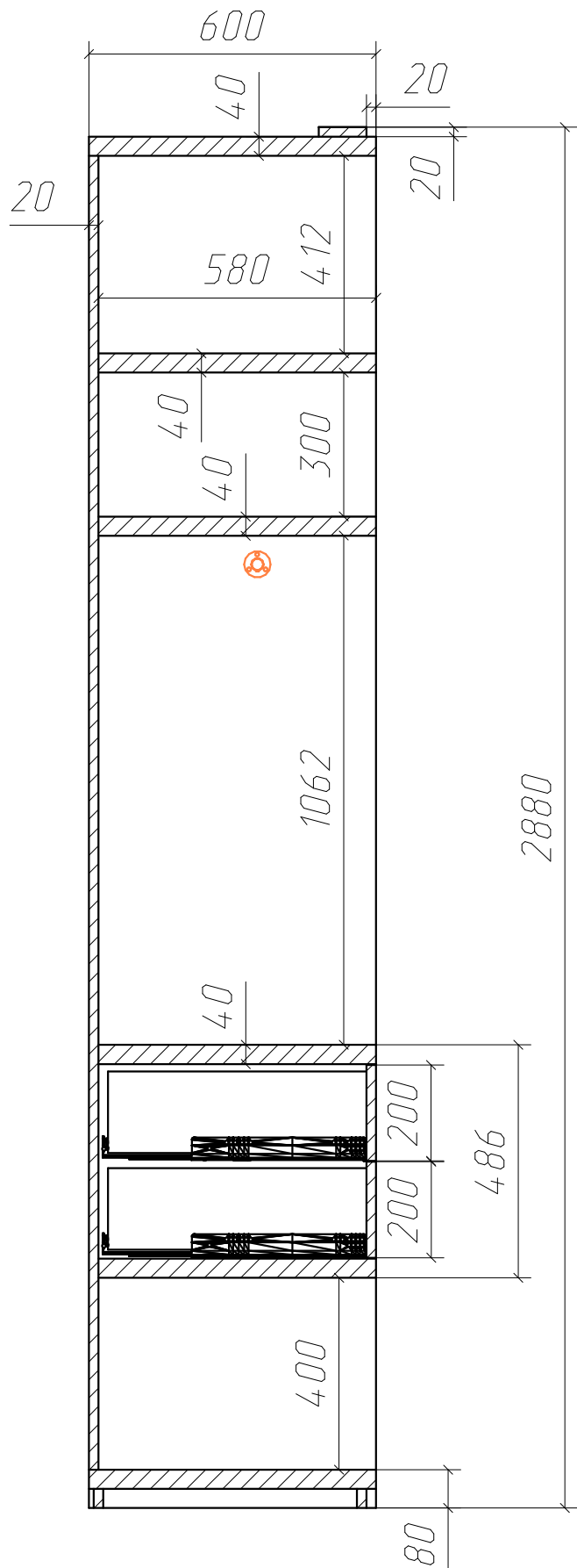
Сечение С-С
