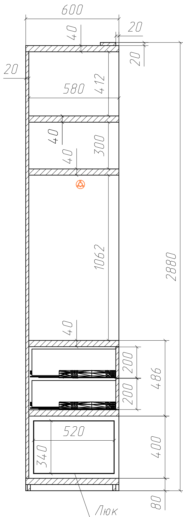
Сечение D-D
