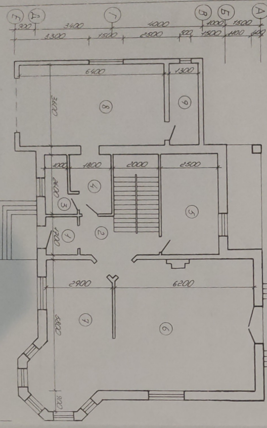
ПЛАН 1-го ПОВЕРХУ
