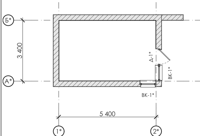
План поверху М1:100
