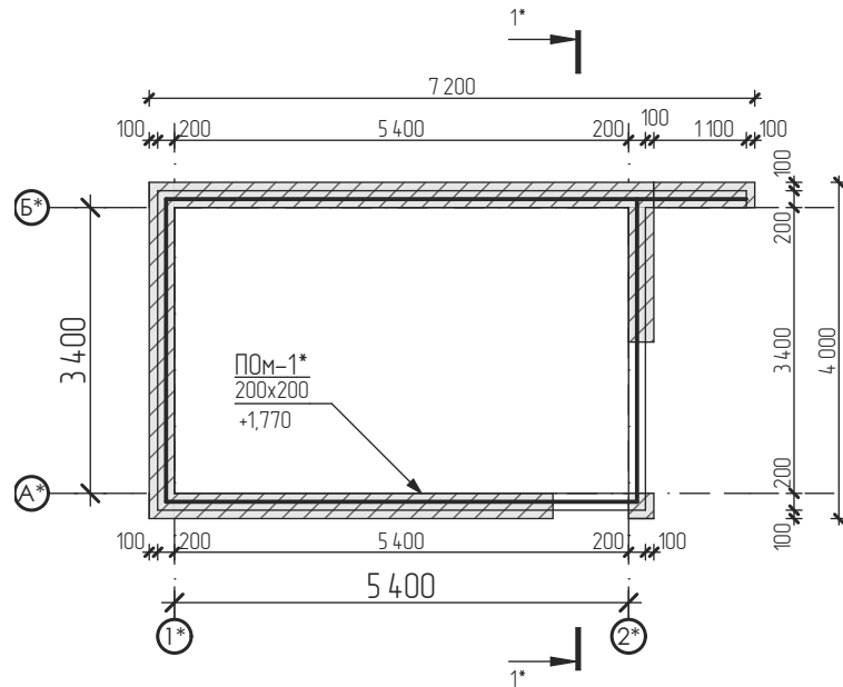
Схема монолітного поясу на відм.+1,770 М1:100
