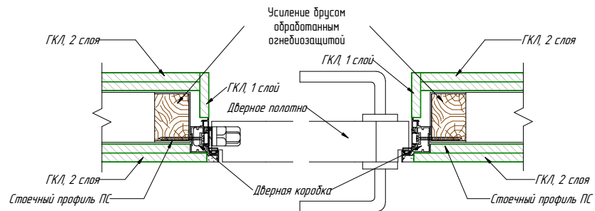
Типовой узел монтажа дверной коробки с усилением проема (в проем)
