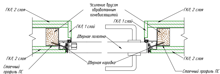
Типовой узел монтажа дверной коробки с усилением проема (из проема)
