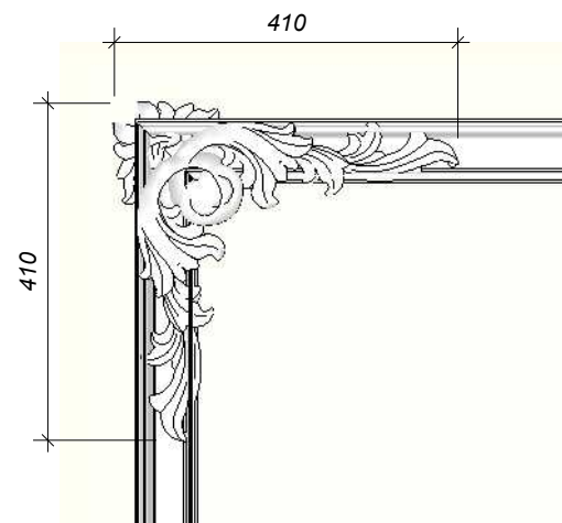
К1-25.0м/п
