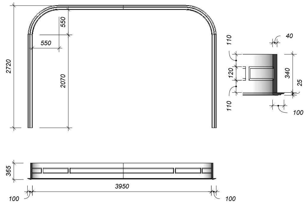
Оздоблення стіни в приміщенні №124
