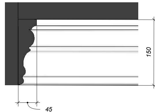
К2-20.0м/п
