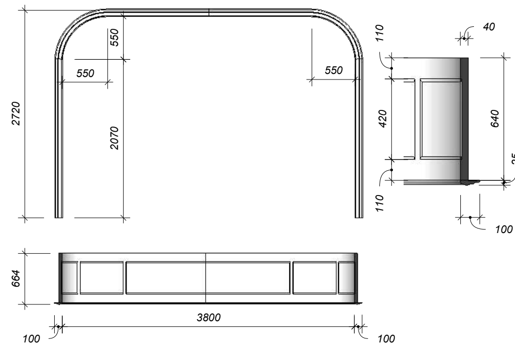
П 2-1шт
