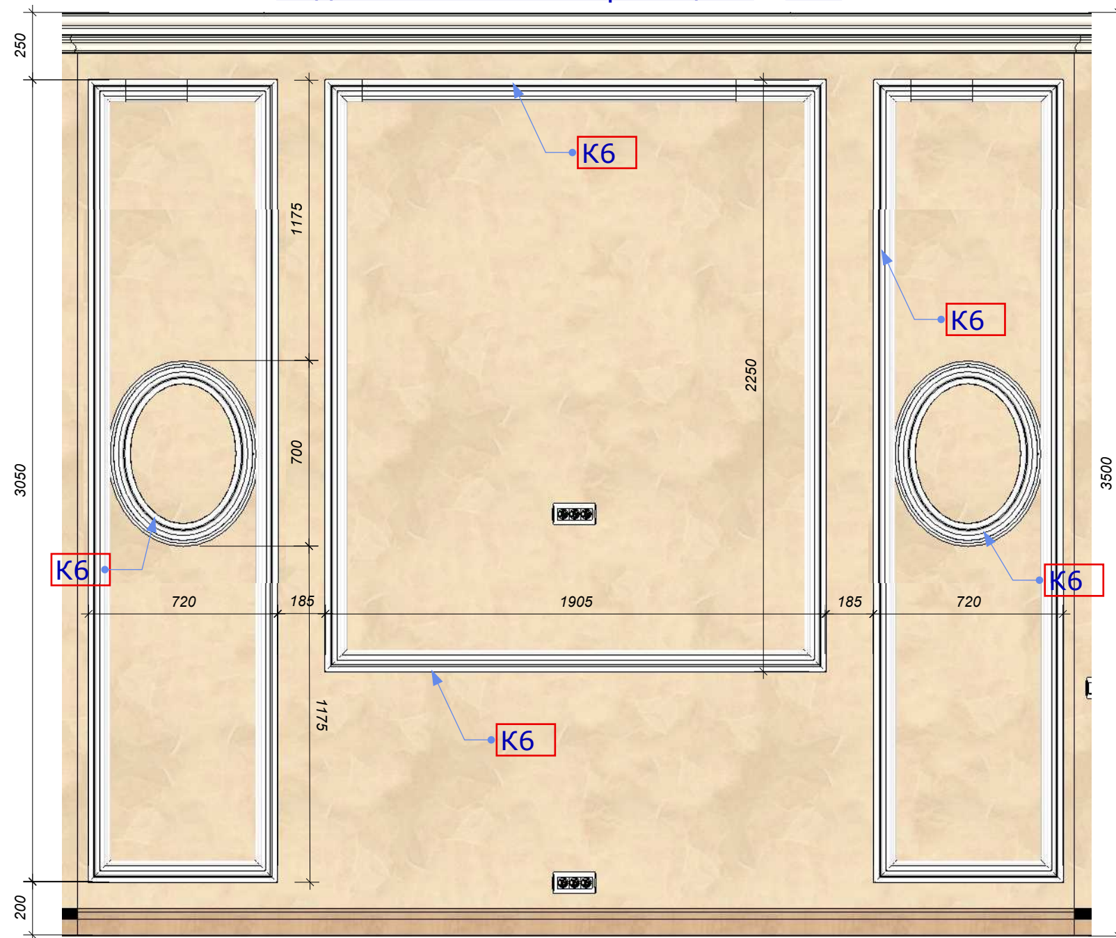
Оздоблення стіни в приміщенні №124
