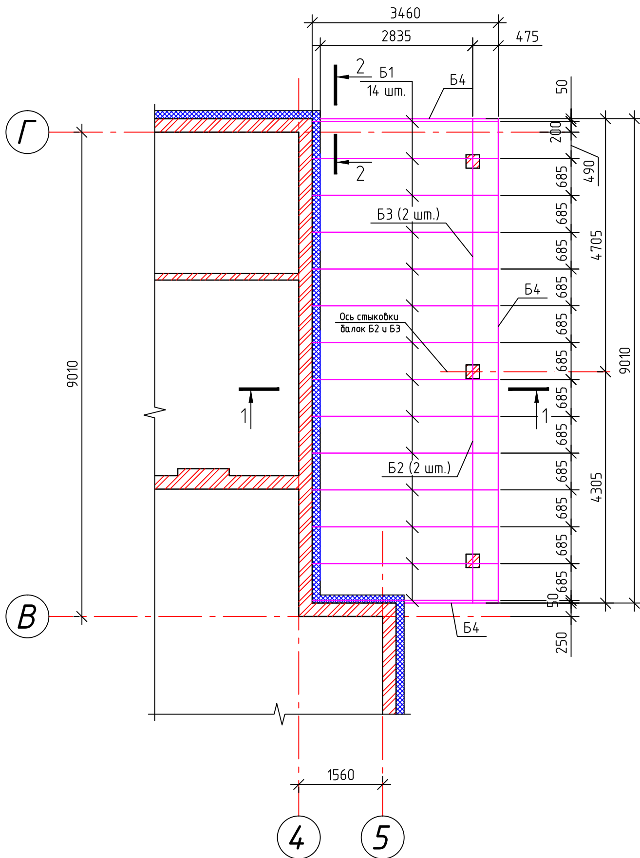
План стропил навеса террасы
