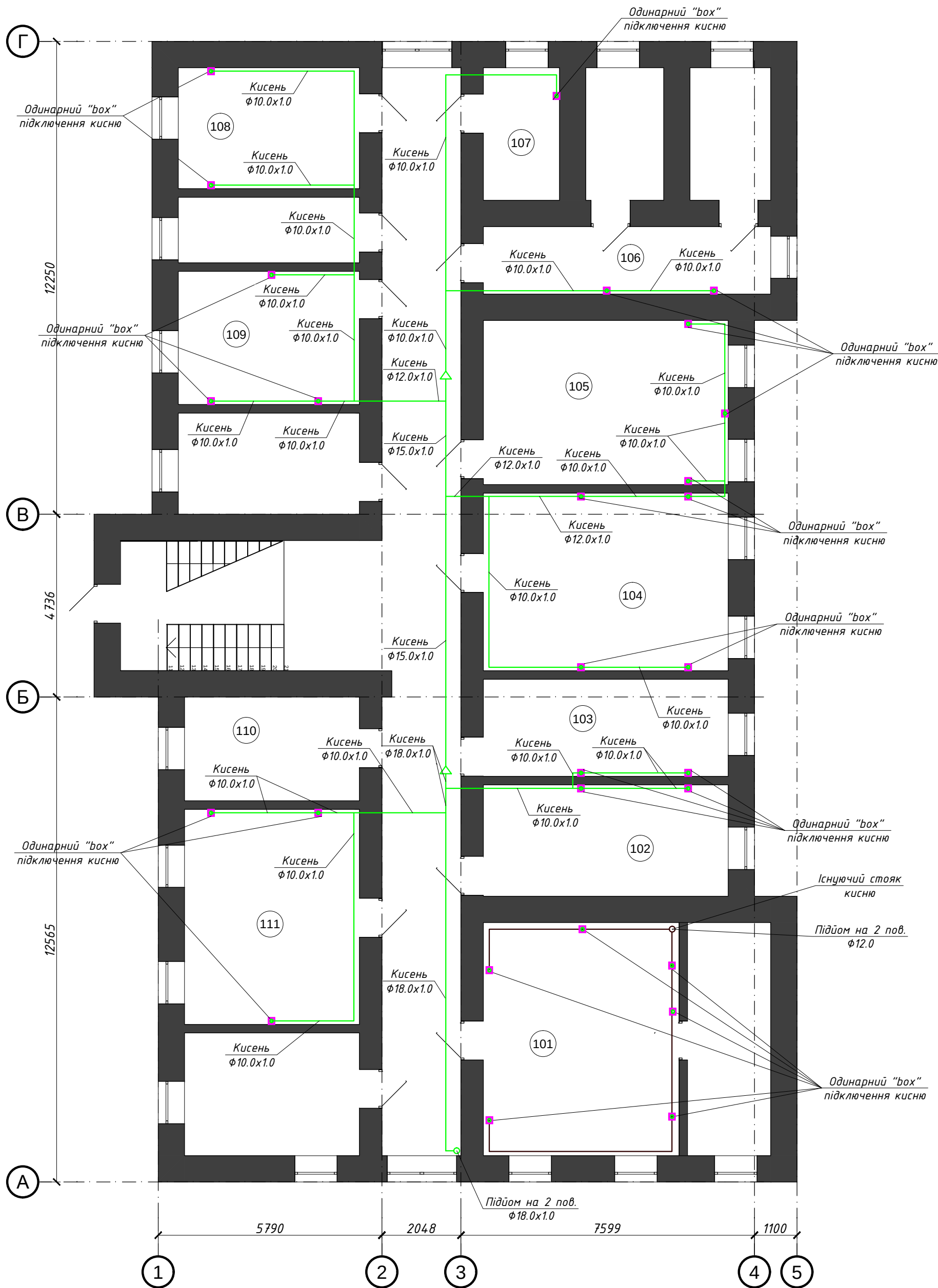
Інфекційний корпус. План 1-го поверху (Палати COVID-19)
