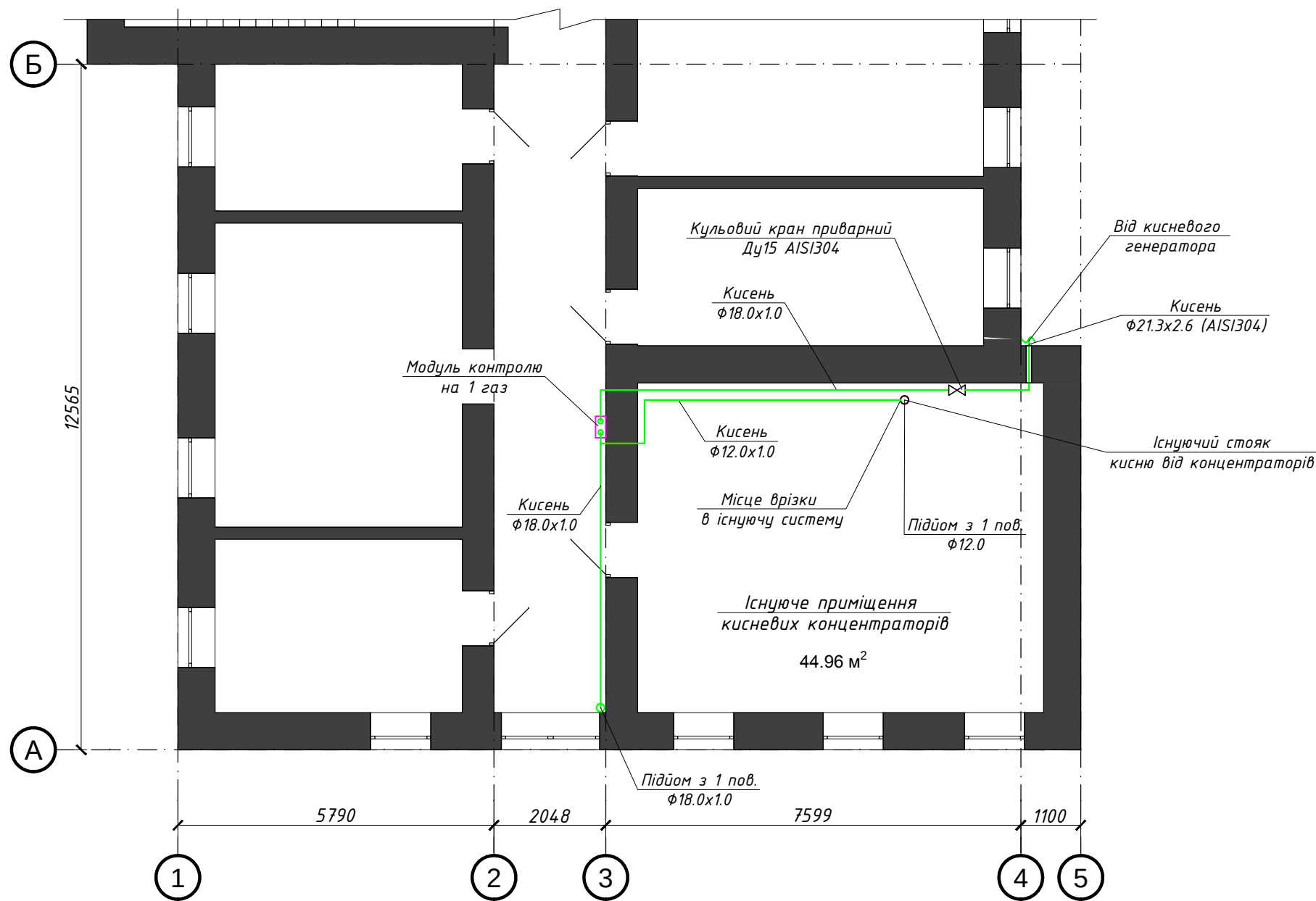
Інфекційний корпус. Фрагмент плану 2-го поверху
