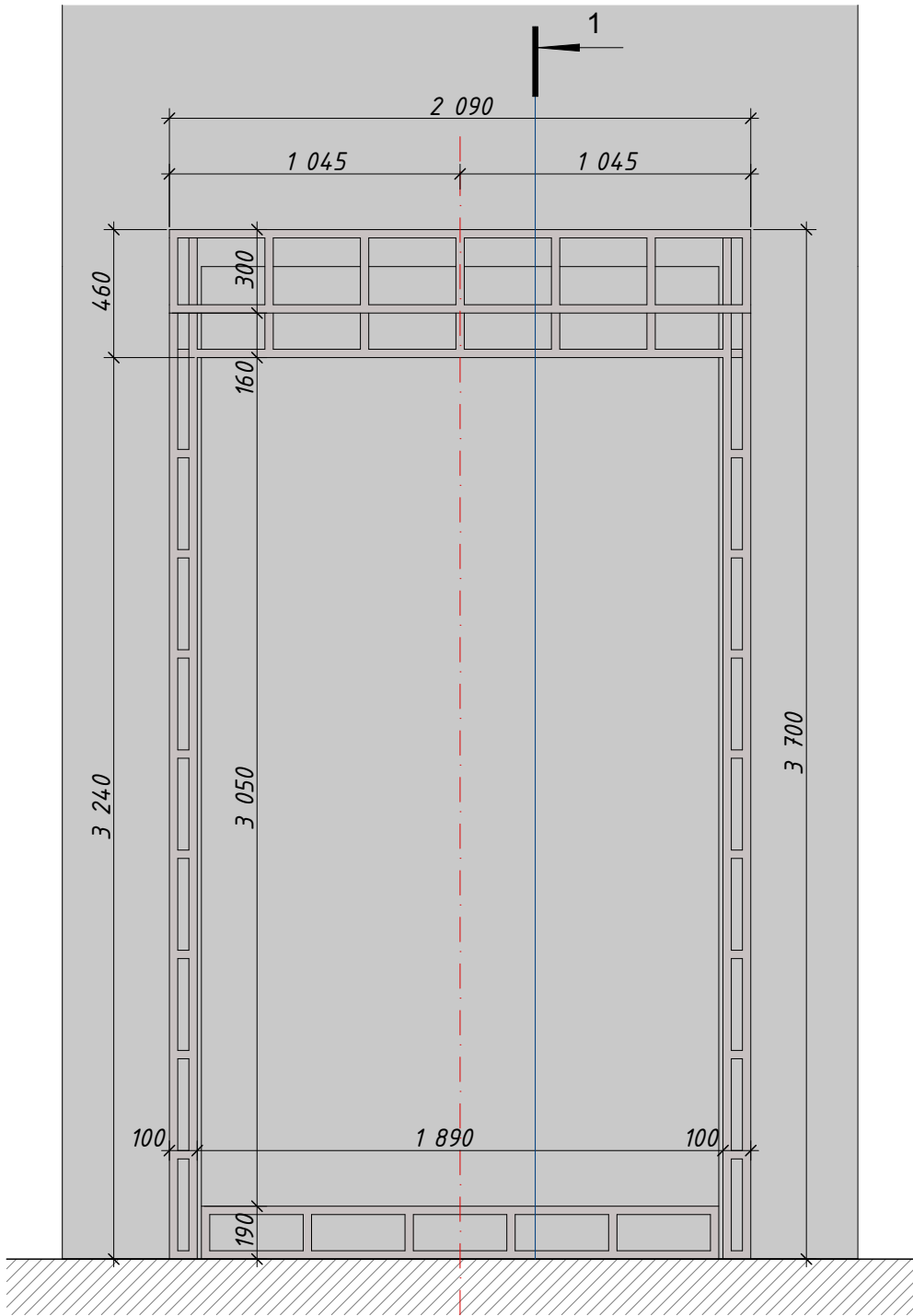
Фронтальний вид
