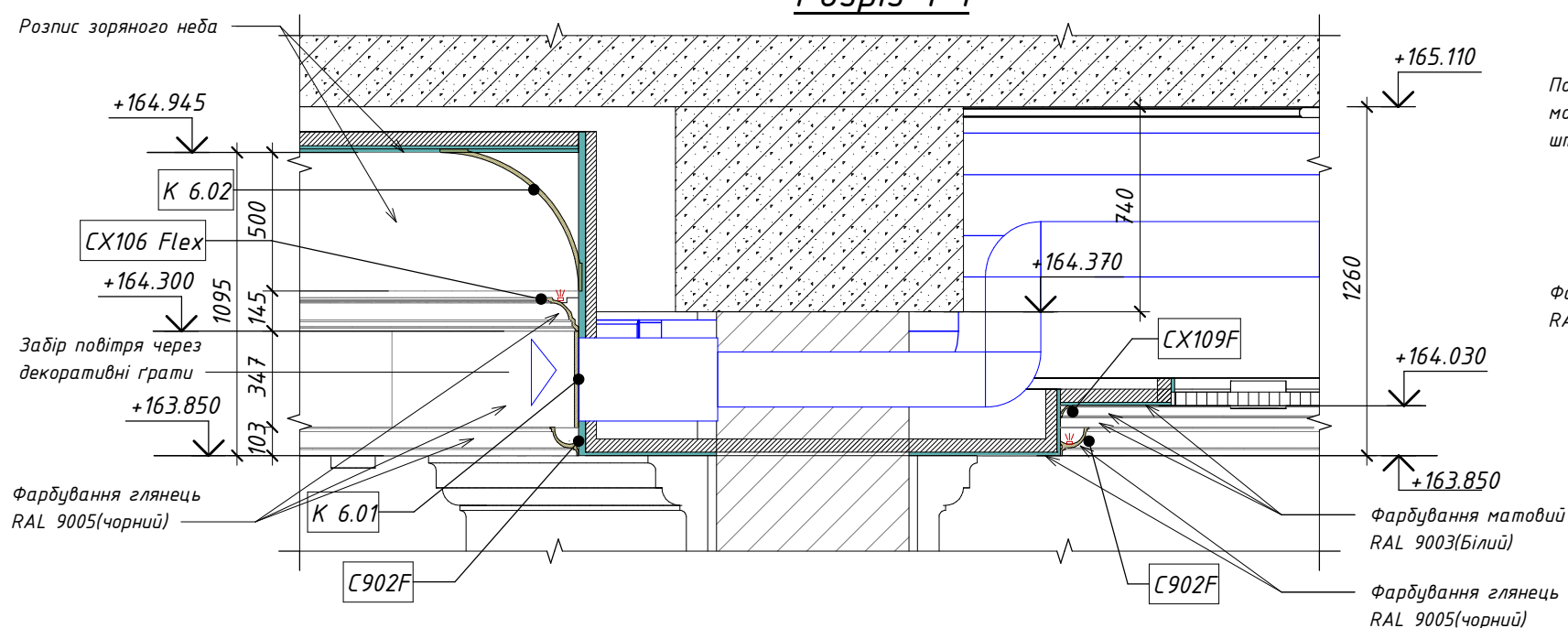
Розріз 1-1
