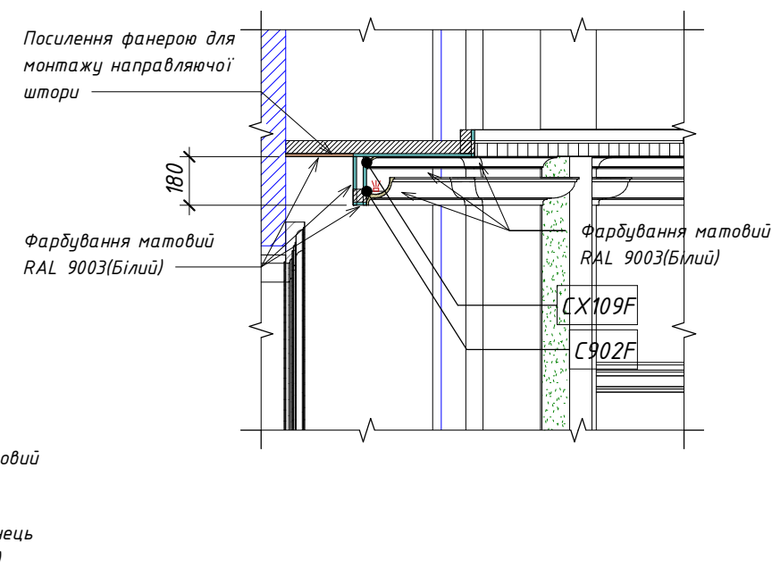
Розріз 2-2
