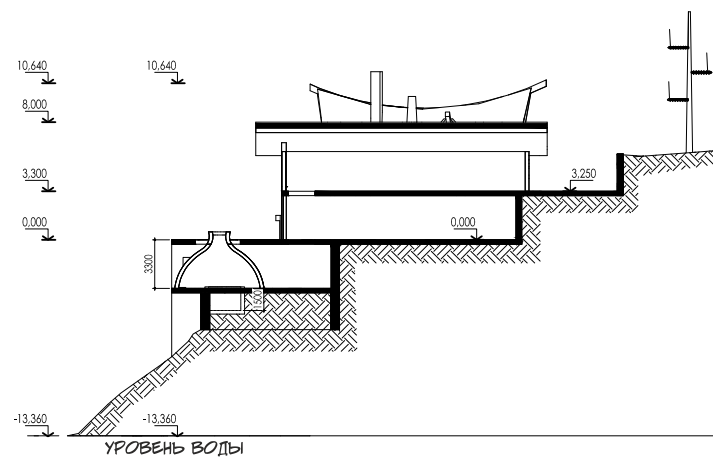
РАЗРЕЗ 2-2
