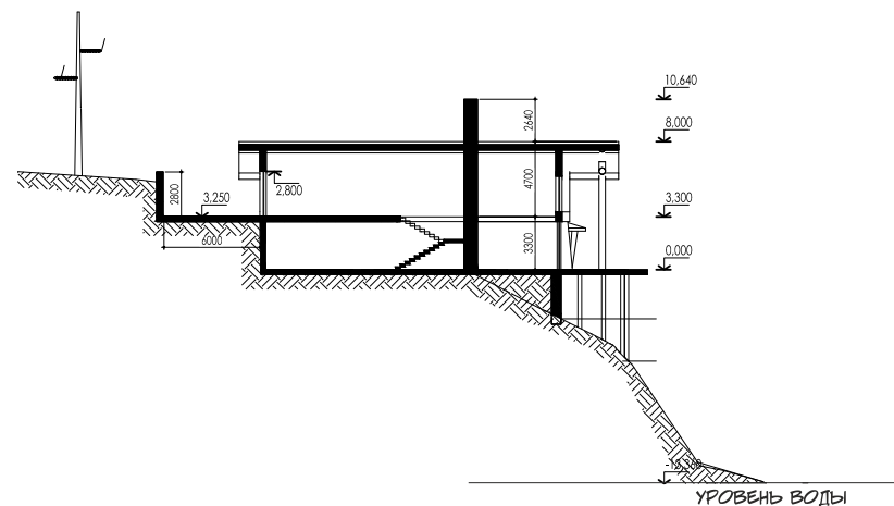
РАЗРЕЗ 3-3
