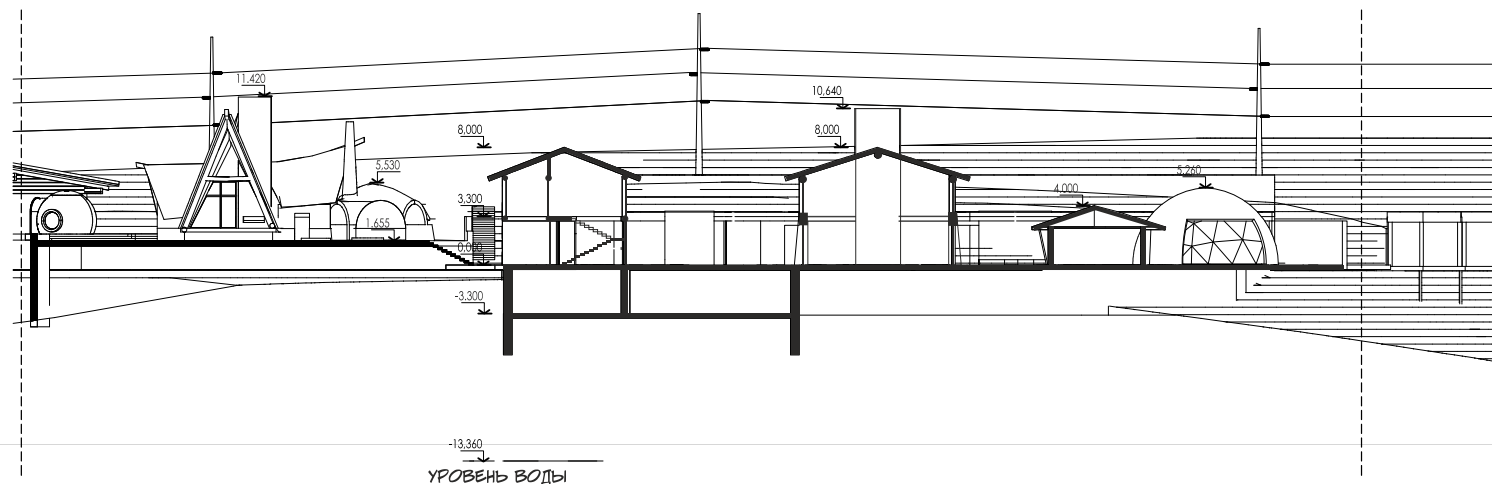
РАЗРЕЗ 1-1
