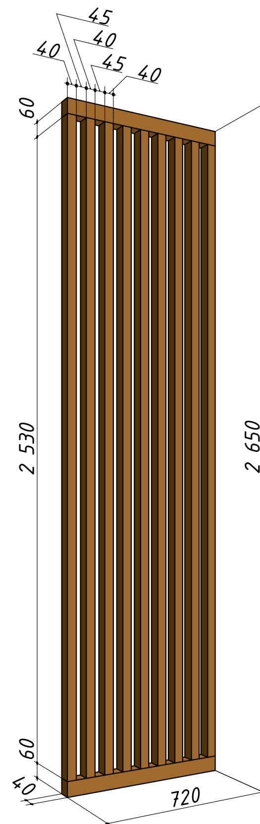
Розміри секції розсубної перегородки
