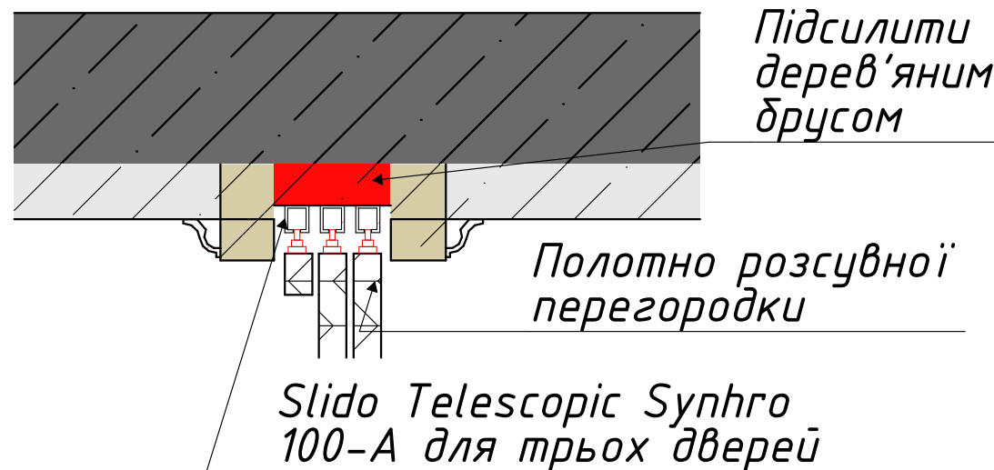
Розріз розсубної перегородки
