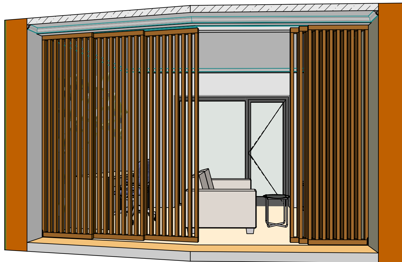
Розріз розсубної перегородки
