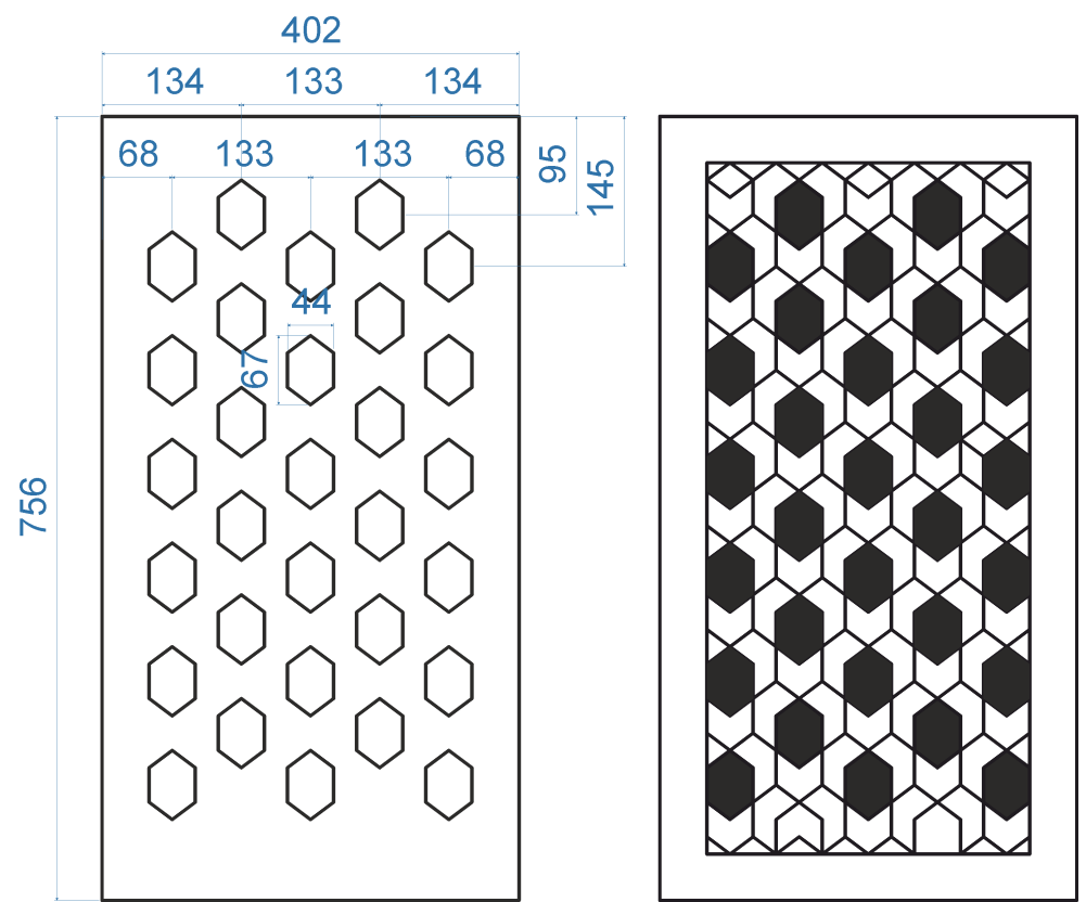
Фрезерування фасада під кошик для білизни
