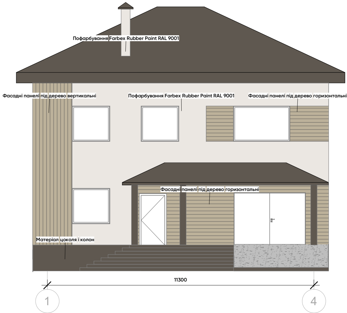
Фасад в осях 1-4
