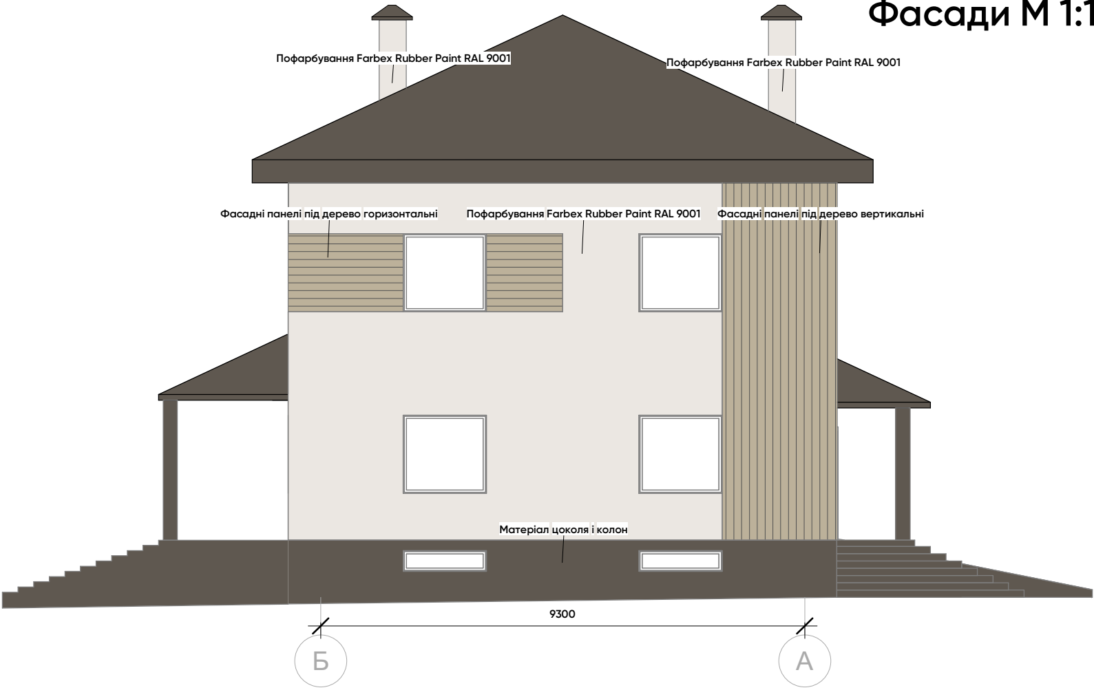
Фасад в осях Б-А
