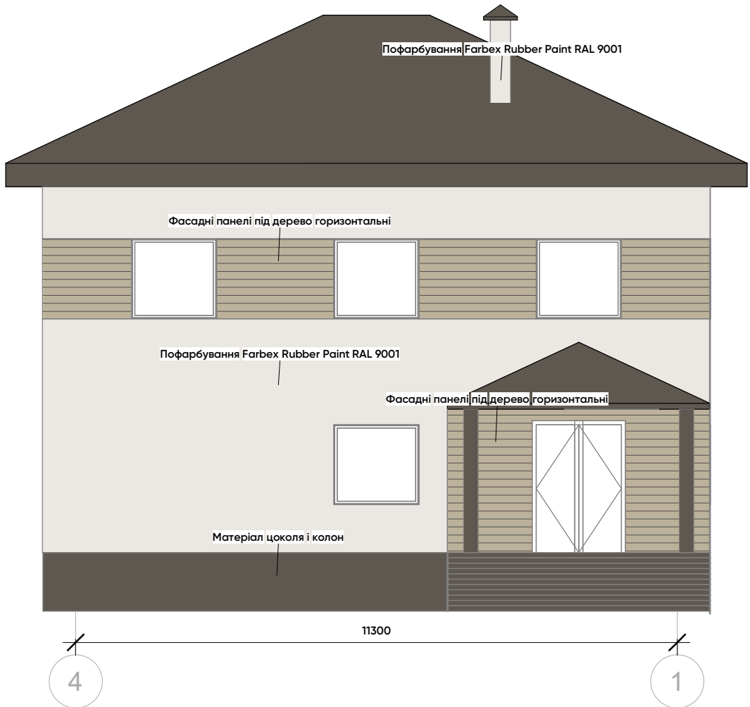
Фасад в осях 4-1
