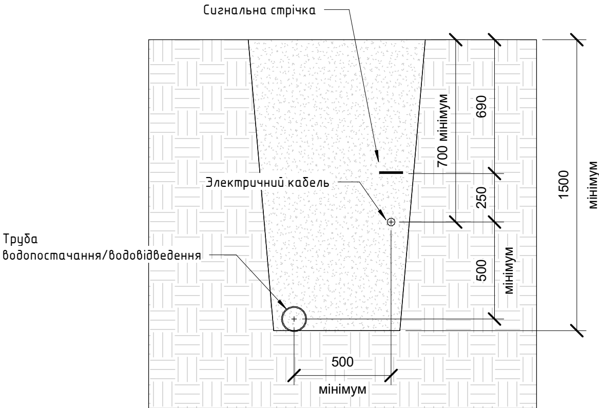
СХЕМА ТРАНШЕЇ
