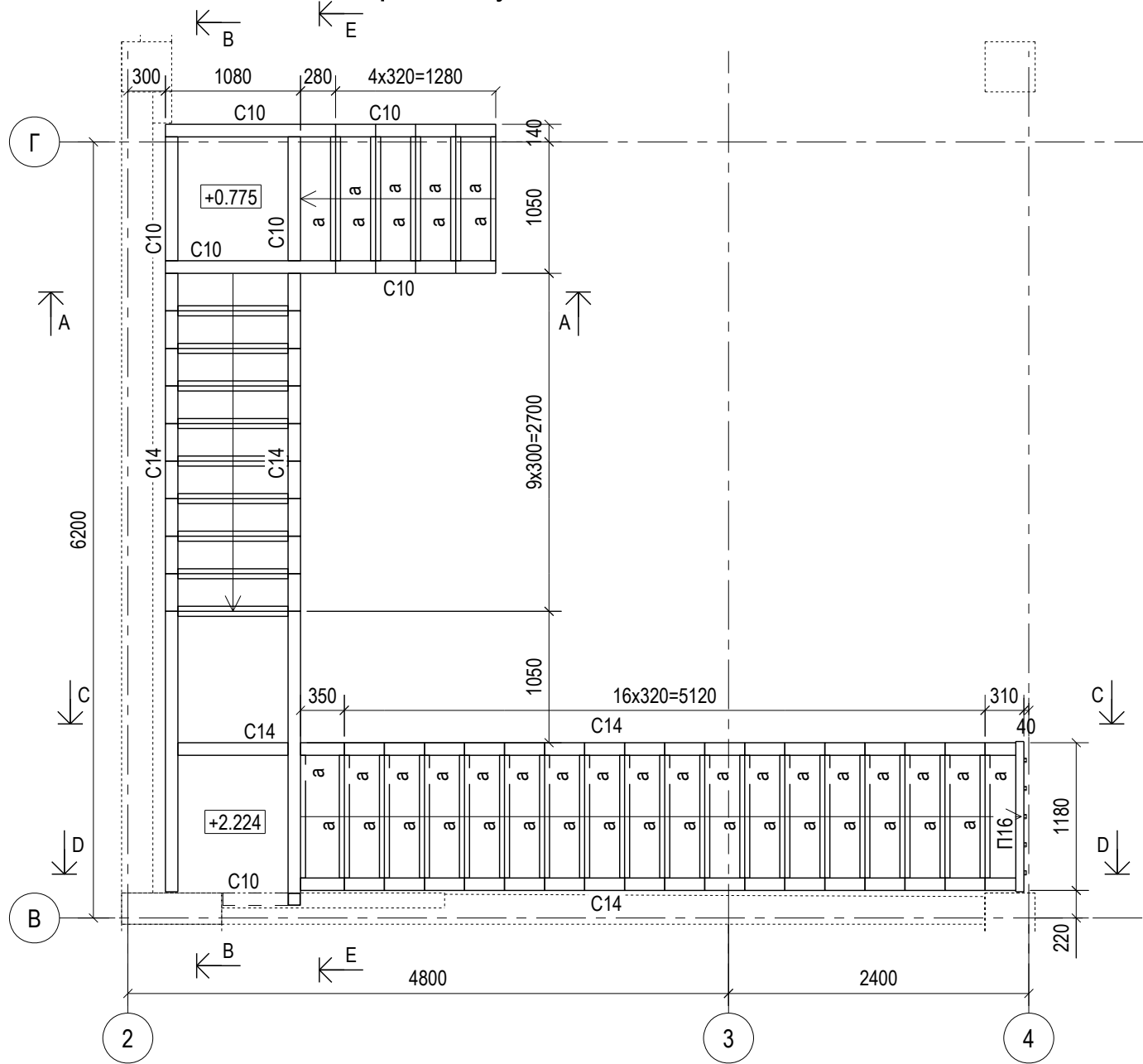
Схема розташування сходів в осях 2-4хВ-Г
