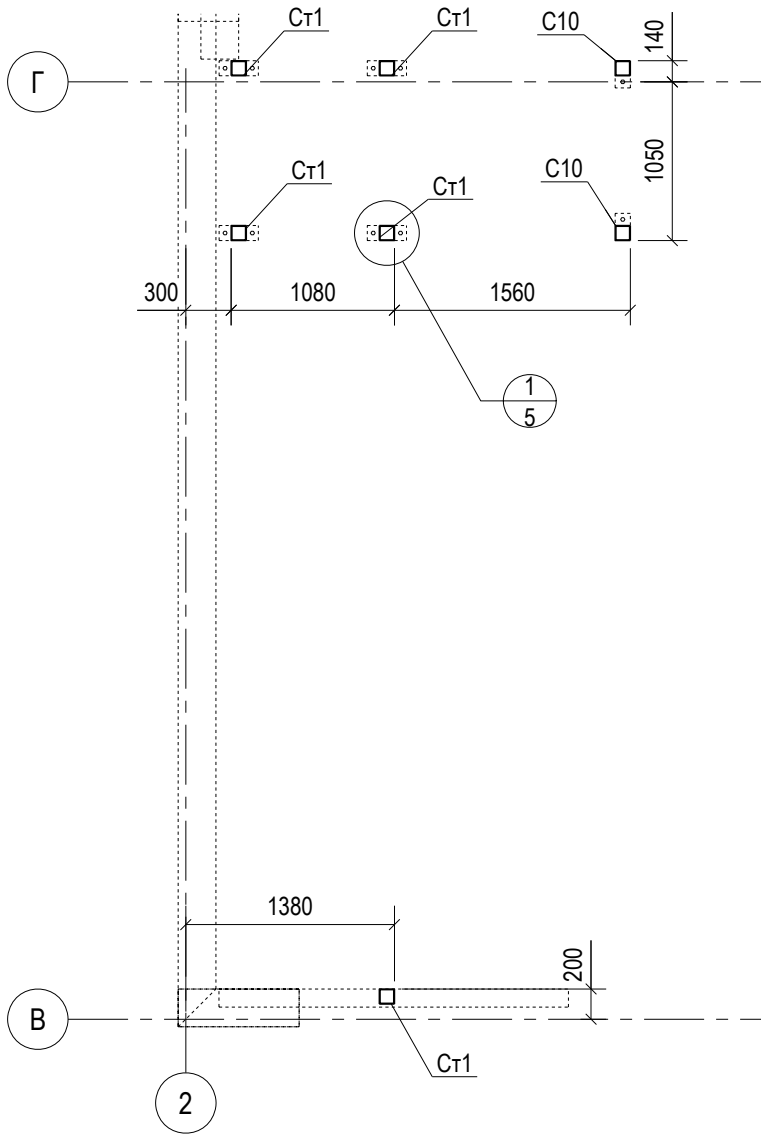
Схема елементів на відм. 0.000
