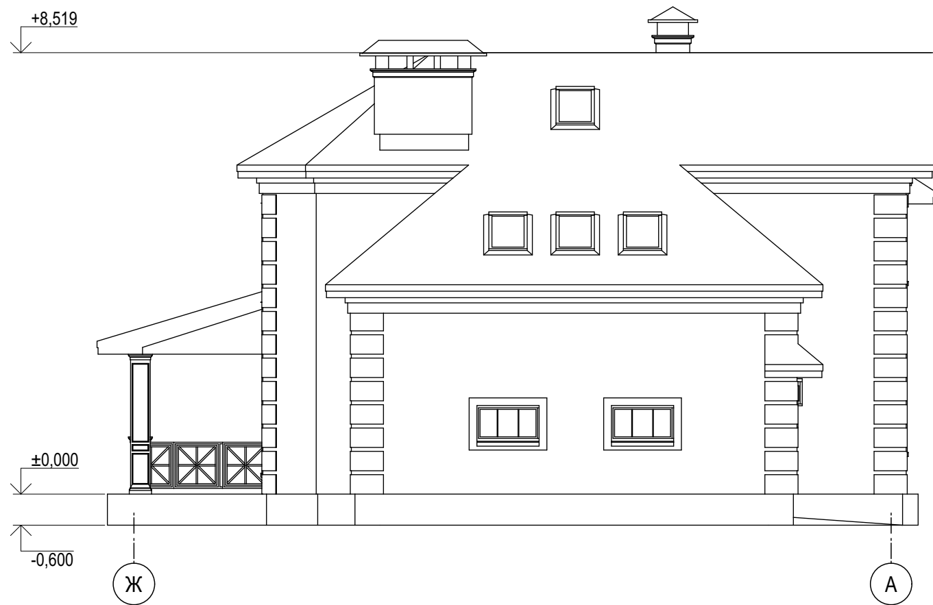
Фасад у вісях Ж-А
