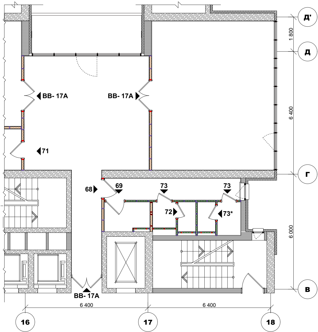
Специфікація заповнення дверних прорізів
