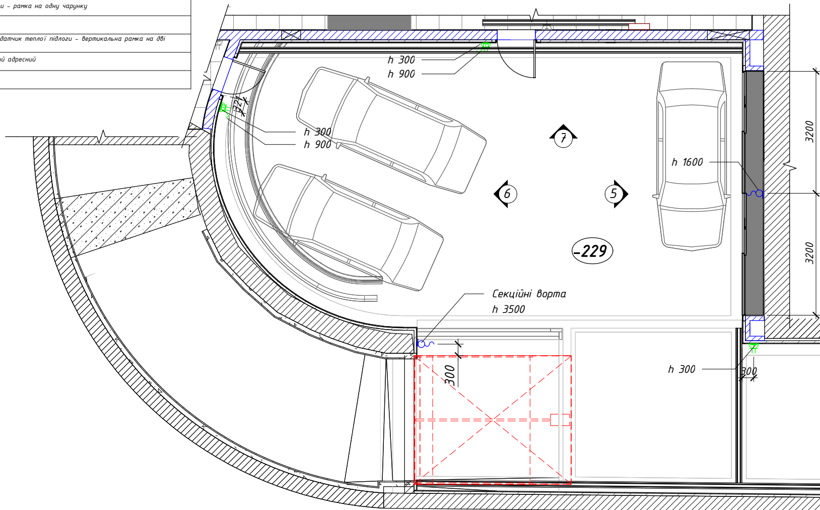
Фрагмент 1. План
