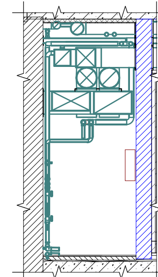
Розгортка 2
