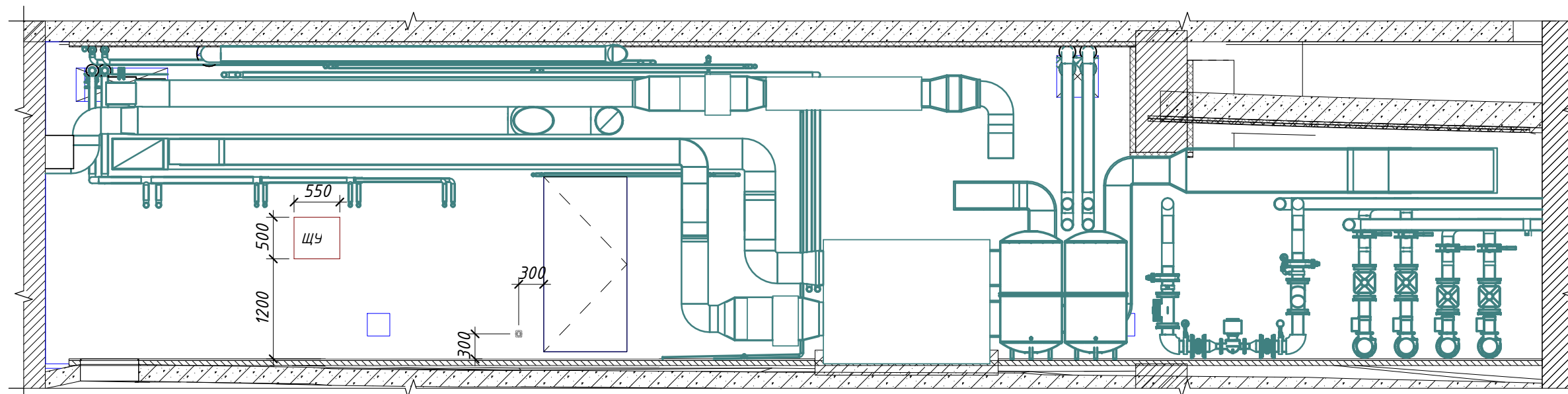
Розгортка 3
